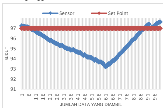
Gambar 4.4 Data perubahan sensor ketika diberi gangguan kearah kanan
