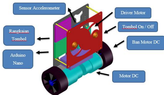
Gambar 3.1. Perencanaan Konstruksi Robot Balancing.
