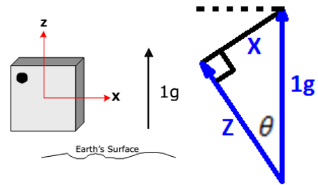
Gambar 2.5 Penempatan sumbu x dan y pada Accelerometer
