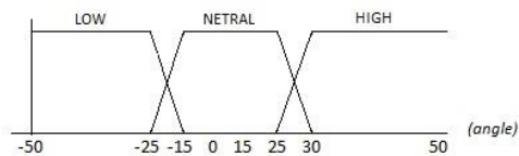
Gambar 2.1 Fungsi keanggotaan
