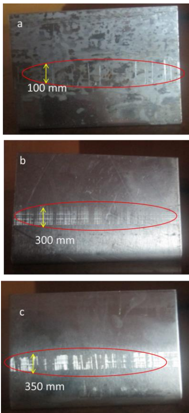
Gambar 6. Stretch mark hasil bending dengan sudut Dies 70°, Plat almunium tebal (a) 1 mm, (b) 2 mm, (c) 3 mm.
