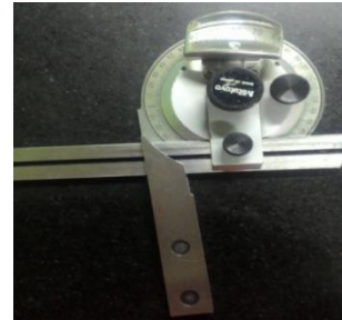
Gambar 3 : Bevel Protactor
