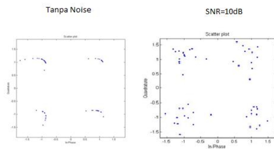
Gambar 9: Scatter diagram setelah Equalisasi
