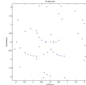
Gambar 8: Scatter diagram QAM-4 melalui kanal b
