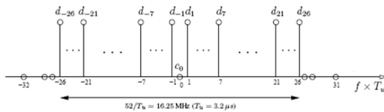
Gambar 4: SC pada 802.11a/g
