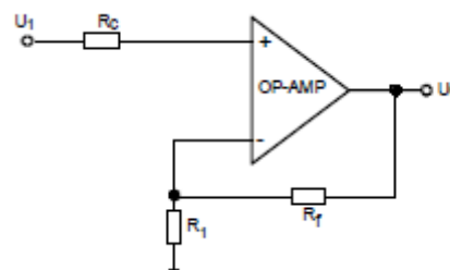
Gambar 2.2 Rangkaian OP-Amp
