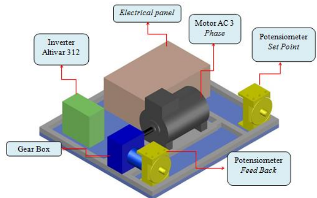
Gambar 3.2 Perancangan 3D
