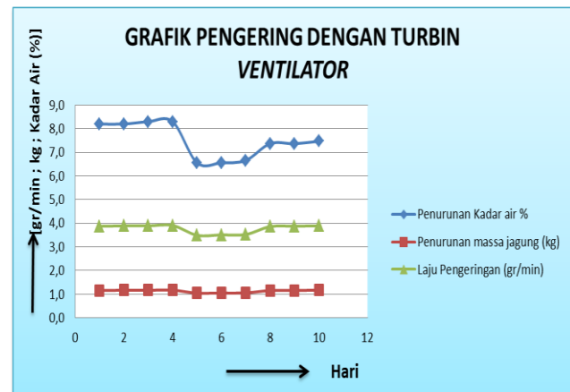
Gambar 5 : Grafik Kadar Air dan Massa Jagung dengan menggunakan Turbin Ventilator
