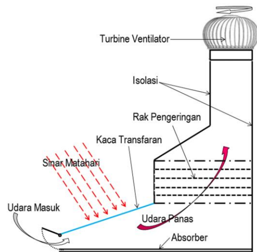
Gambar 1 : Alat Pengering
