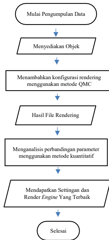
Gambar 3.1 Tahapan Penelitian
