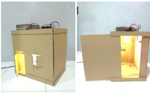
Gambar 4. Rancangan mekanikal pada saat pengujian lampu menyala
