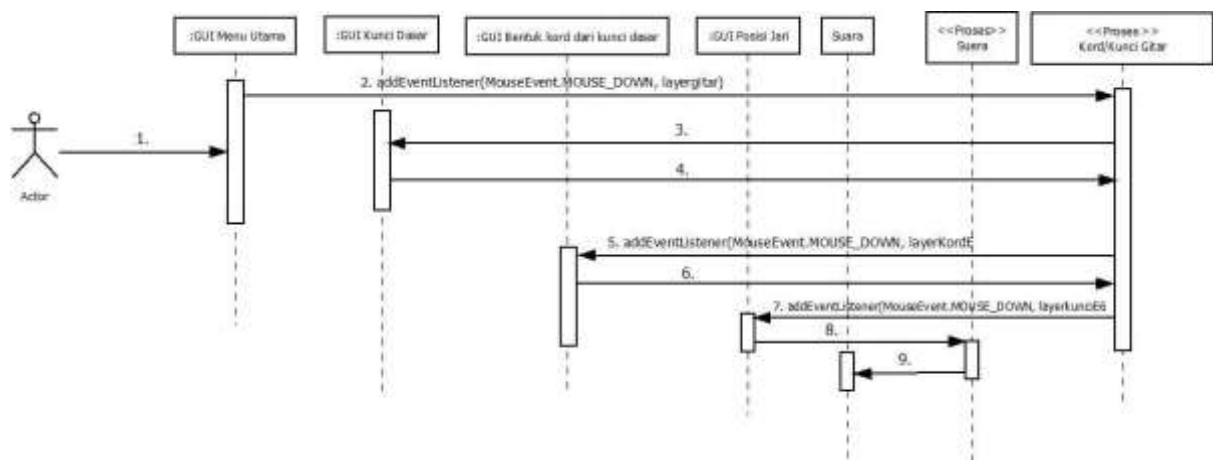
Gambar 7 Sequence Diagram Dengar Kord Gitar
