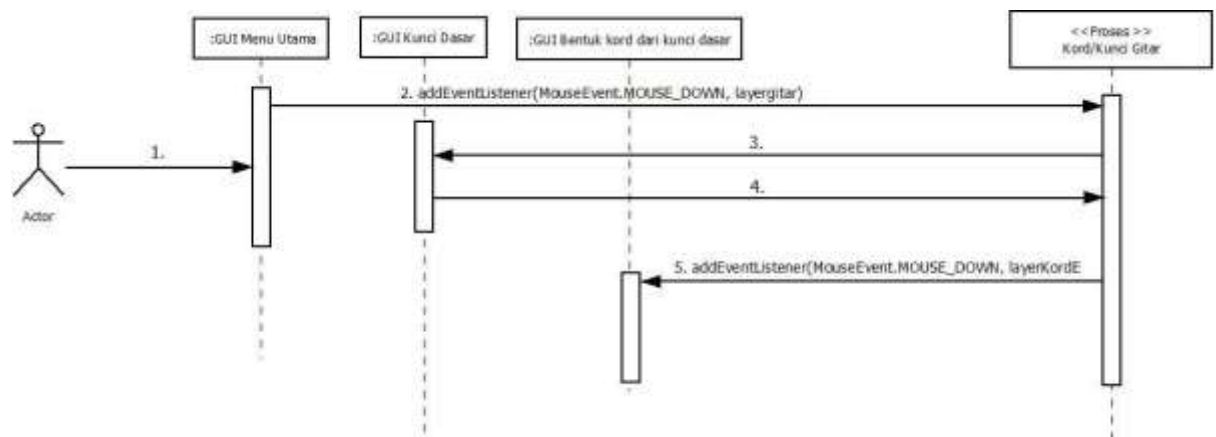
Gambar 5 Sequence Diagram Pilih Kord Gitar
