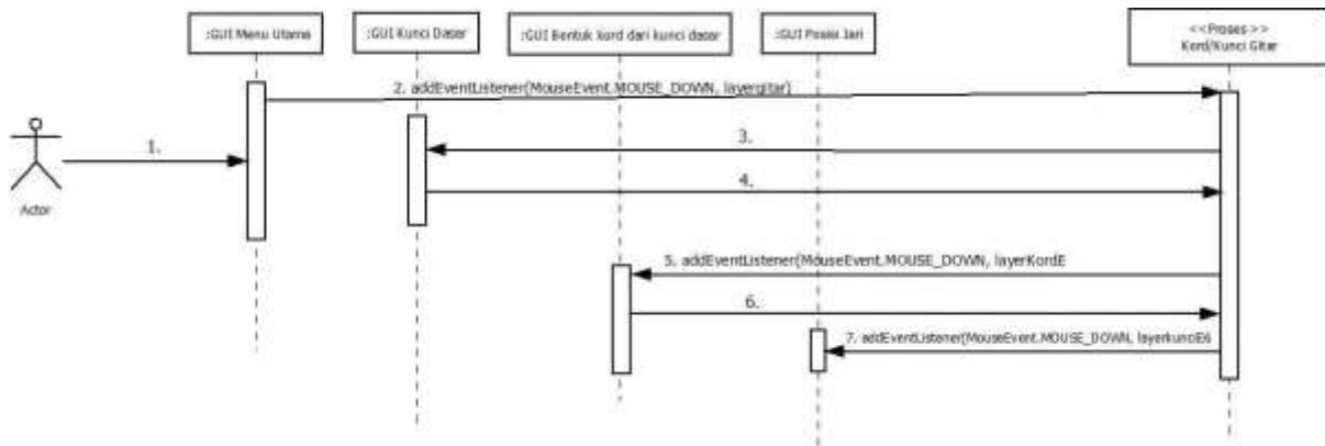
Gambar 6 Sequence Diagram Tampil Kord Gitar dan Posisi Jari
